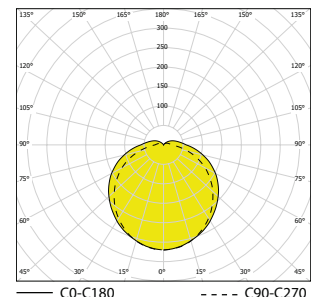
BASET-N-LED-1R
