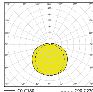
BASET-N-LED-2R
